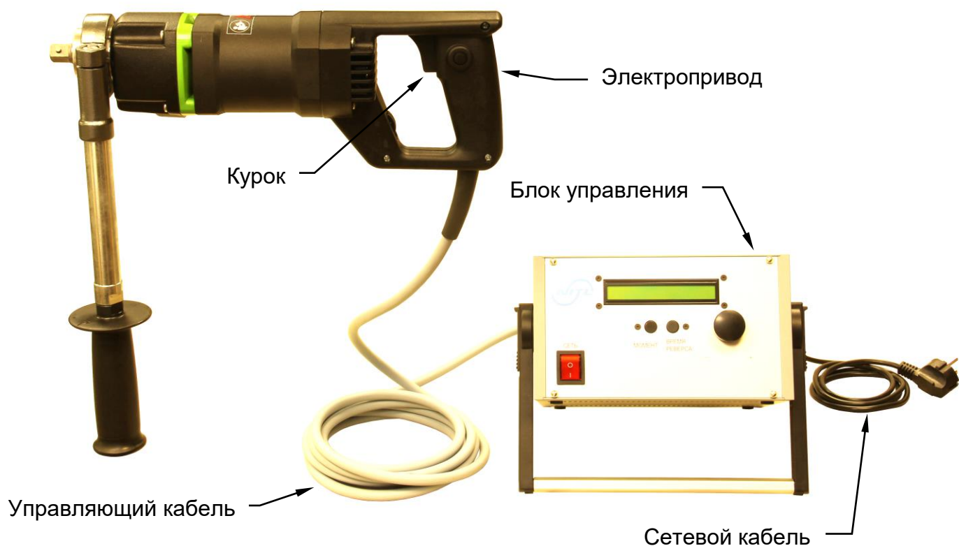
Рис. 1 Общий вид машины
